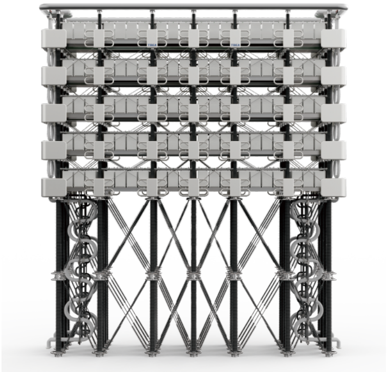
±800kV/8GW高端阀塔图
